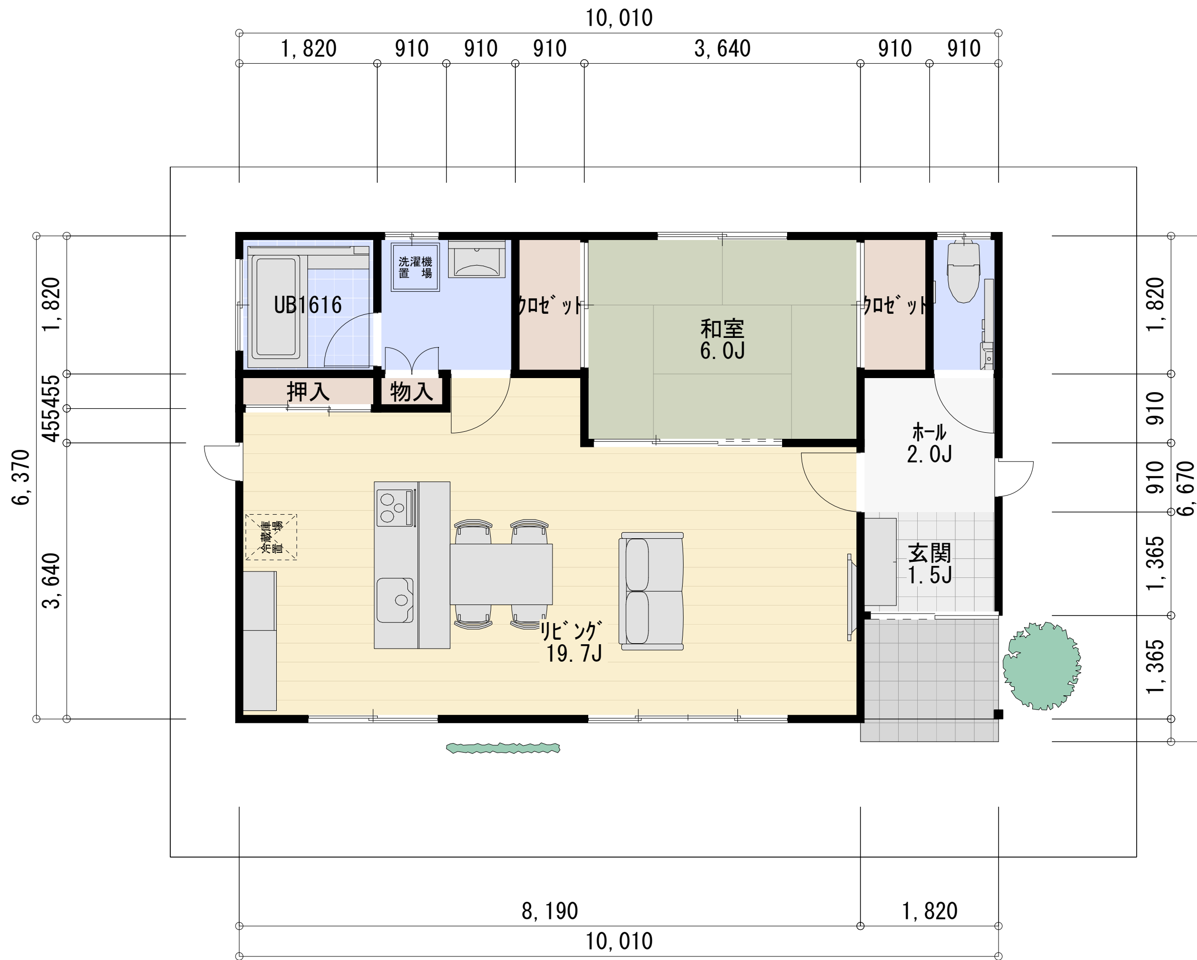
1F平面図
